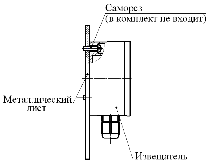
Рисунок 2.4 – Крепление извещателя на металлическом листе
