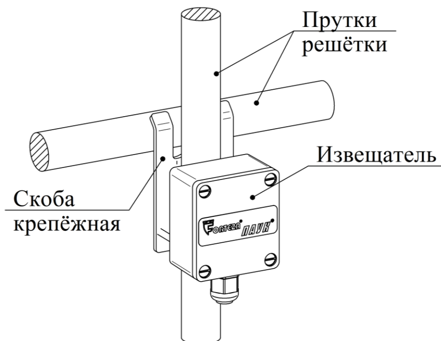
Рисунок 2.1 – Крепление извещателя на решетке из прутка
