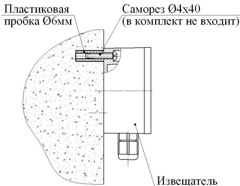
Рисунок 2.7 – Крепление извещателя
