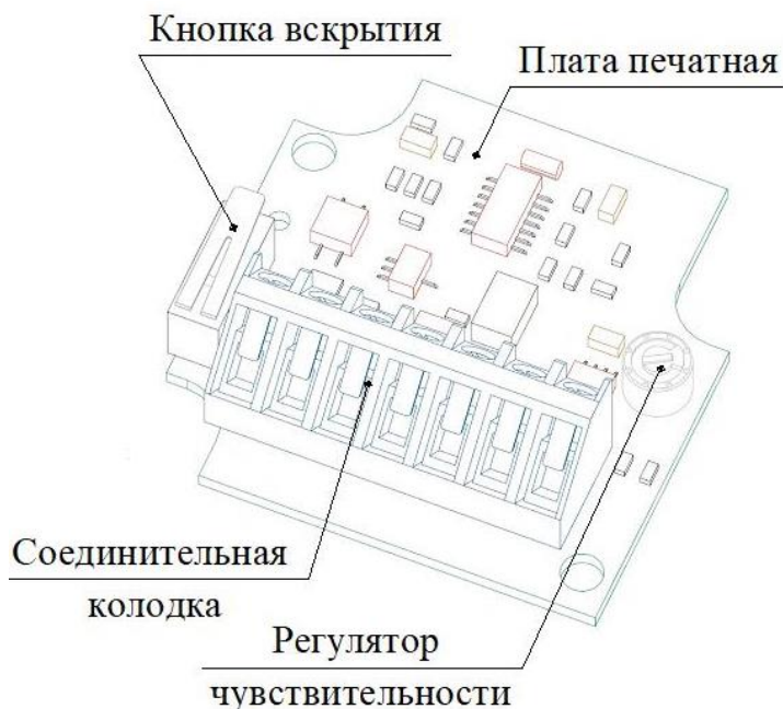
Рисунок 1.2 – Конструкция платы
